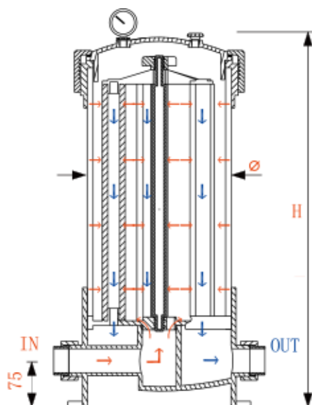
水流示意圖
