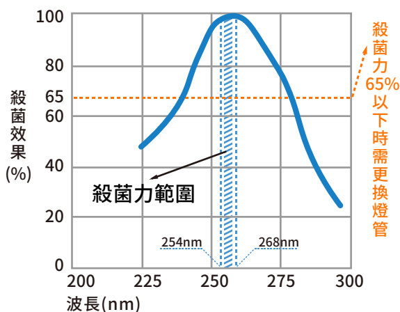
紫外線波長&相對殺菌力曲線圖
